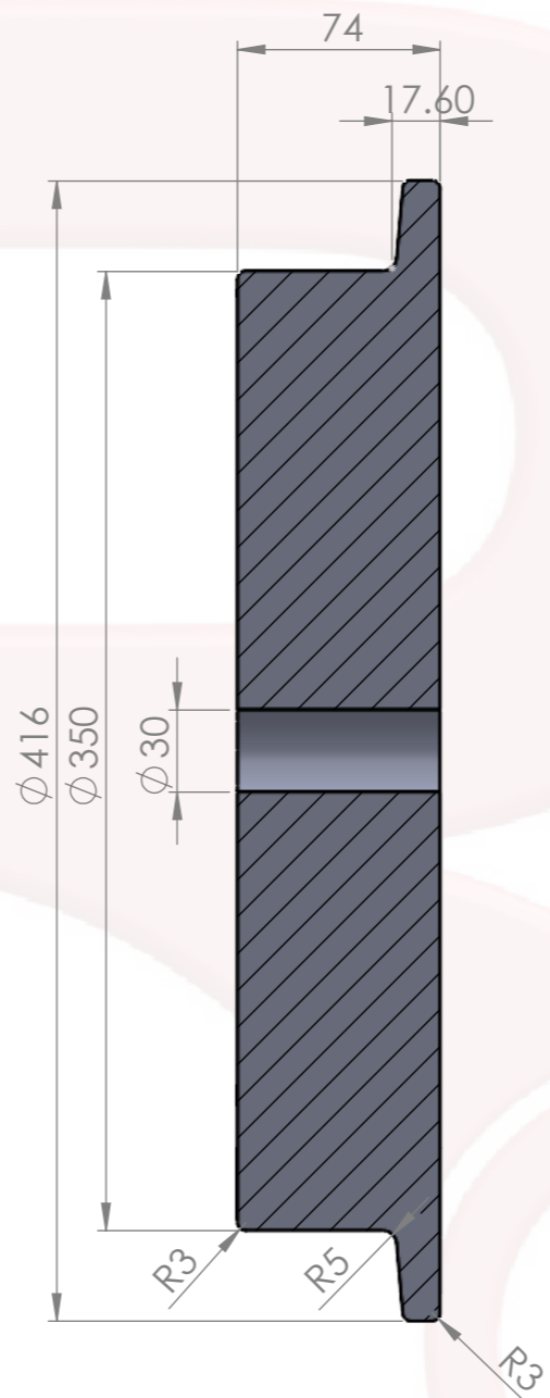
SECTION A-A SCALE 1 : 3
